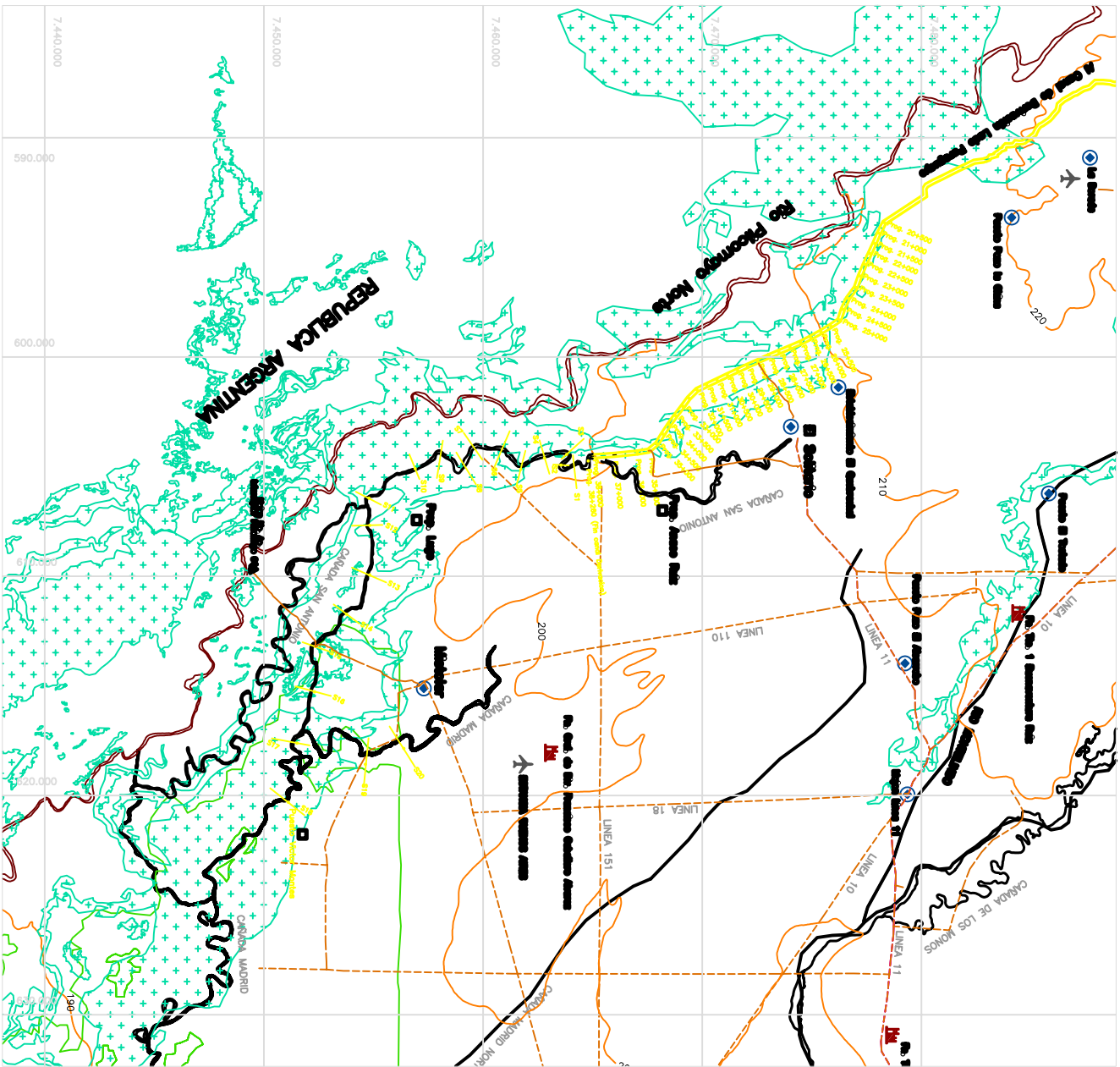
PLANTA GENERAL esc: 1 - 100.000
